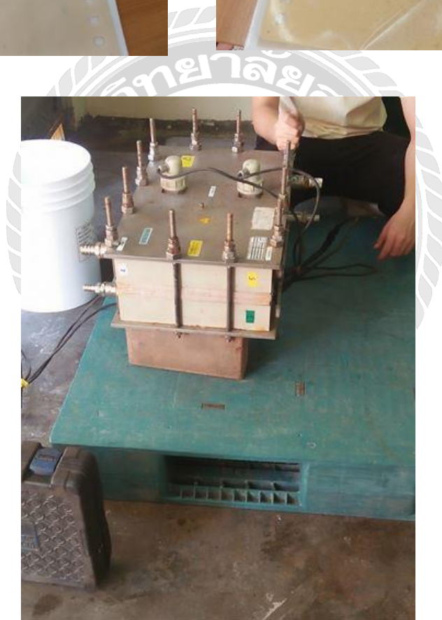
ขั้นตอนการประกอบ membrane stack
