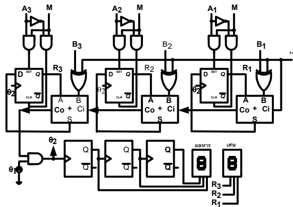
รูปที่ 9 วงจรสมบูรณของวงจรถหารเลขขนาด 3 บิตที่นำเสนอ
