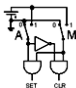
รูปที่ 5 ภาคป้อนอินพุตตัวตั้ง A และ โหมดการเซตค่า M
