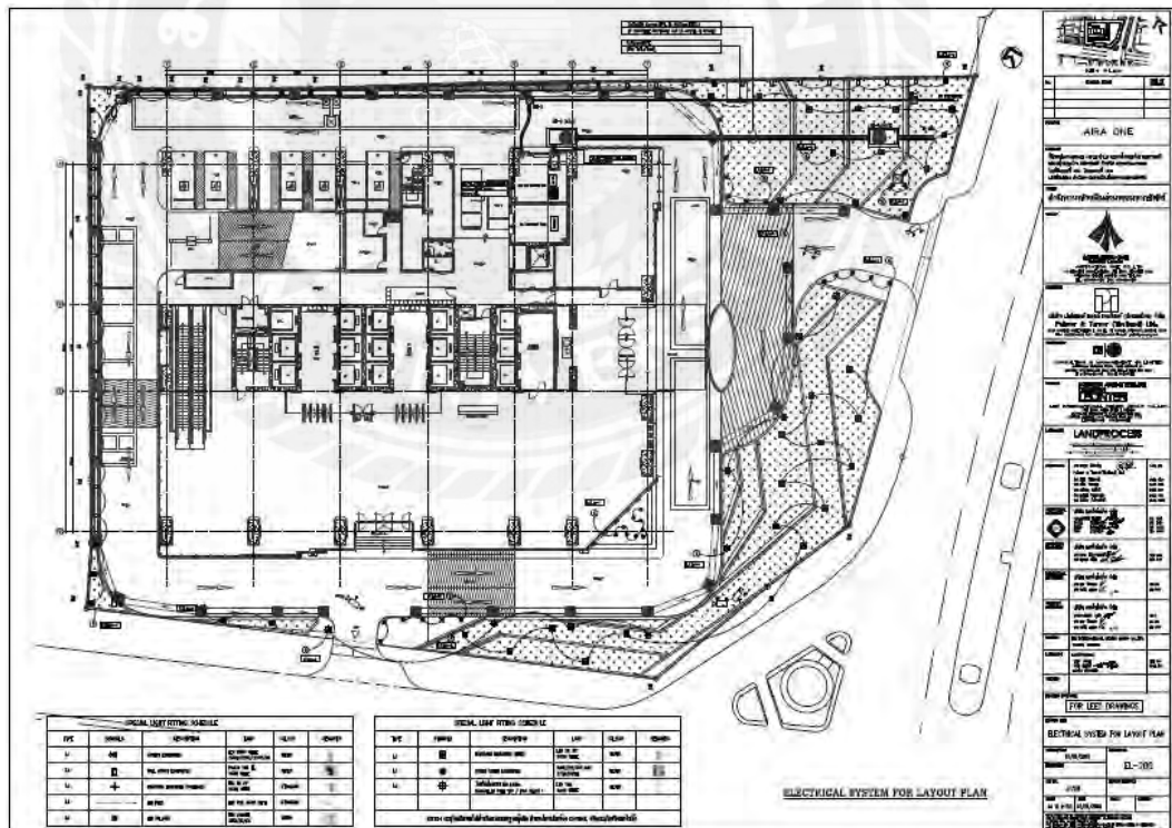
รูปที่ 2 วิธีทางเข้าสายไฟฟ้าแรงสูงและโทรศัพท์มาที่โครงการ
