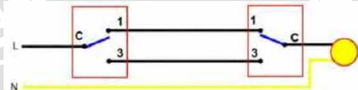
รูปที่ 4.21 ลักษณะการต่อสวิตช์บันไดหรือสวิตช์ 3 ทาง
