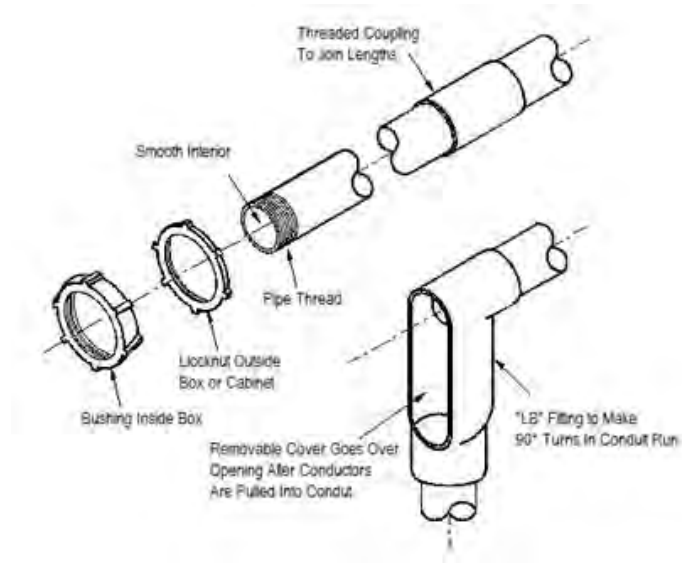
รูปที่ 2.17 การต่อท่อ RMC
