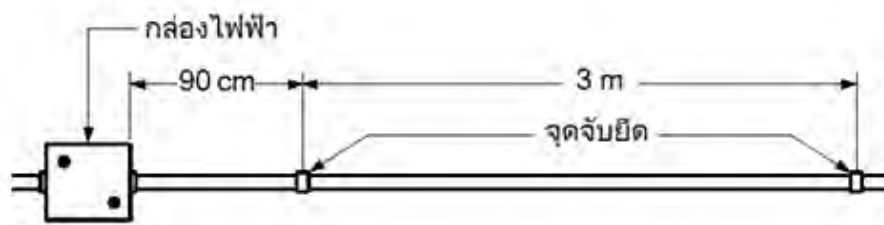
รูปที่ 2.16 การติดตั้งท่อ RMC
