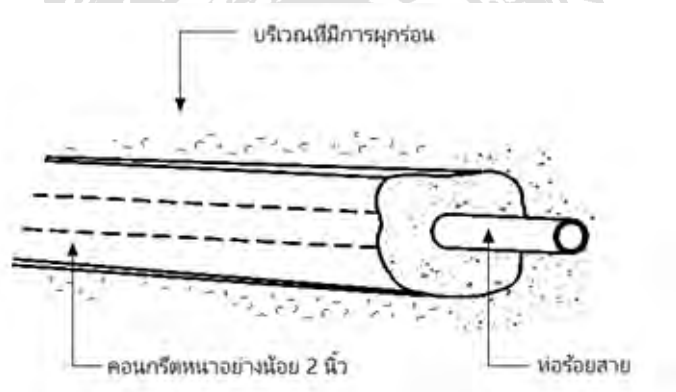
รูปที่ 2.13 การติดตั้งท่อในที่ที่มีการผุกร่อน
