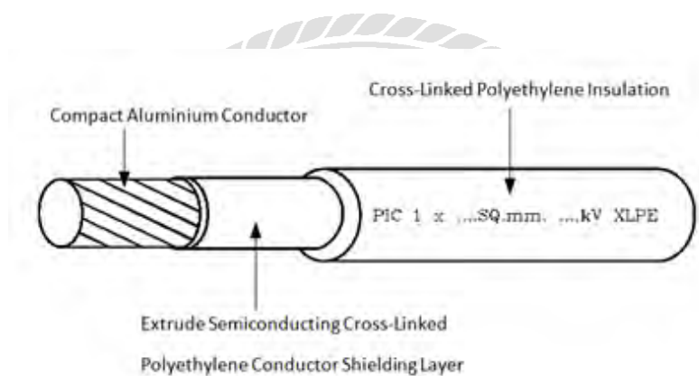
รูปที่ 2.5 สาย PIC
