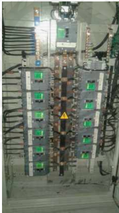
รูปที่ 5 การติดตั้งรางเดินสายไฟเข้าแผงไฟฟ้าย่อย
