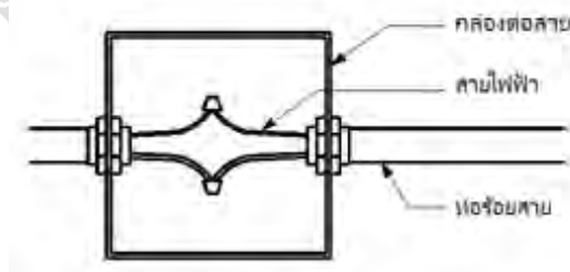
รูปที่ 2.18 การต่อสายไฟ
