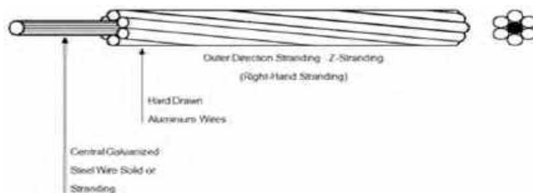
รูปที่ 2.4 สาย ACSR
