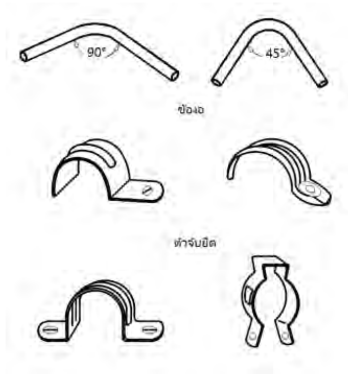
รูปที่ 2.35 ข้องอและตัวจับยึด
