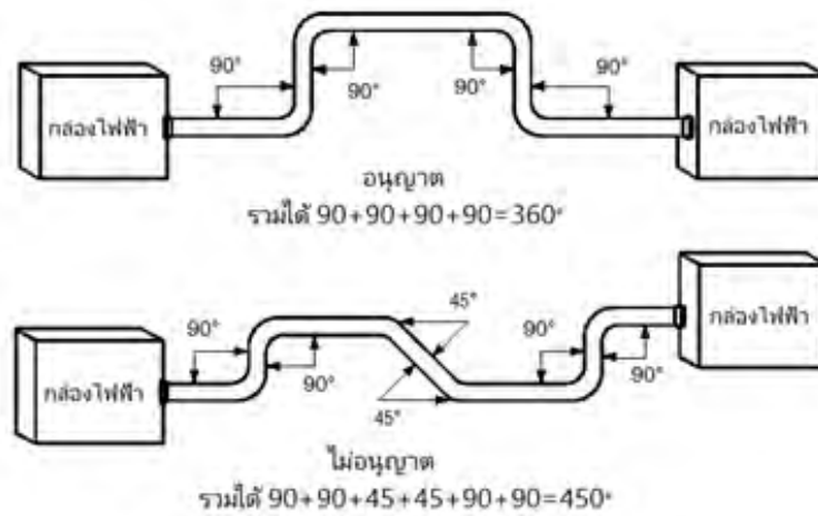
รูปที่ 2.15 มุมตัดโค้งท่อระหว่างจุดดิ่งสาย
