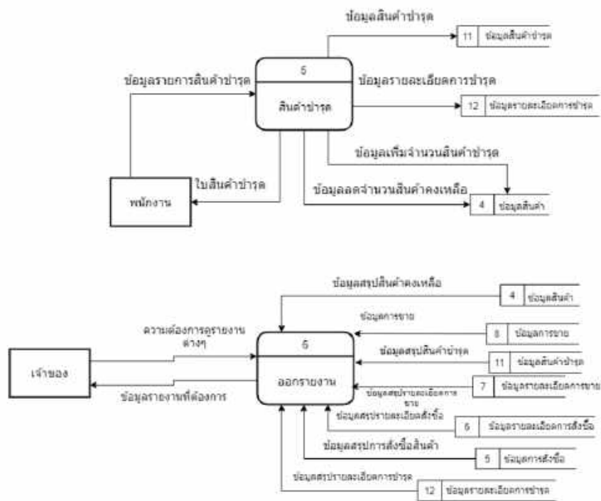
ภาพที่ ก.6 (ต่อ) Data Flow Diagram Level 0 ระบบร้านขายอุปกรณ์การช่าง (ต่อ)
