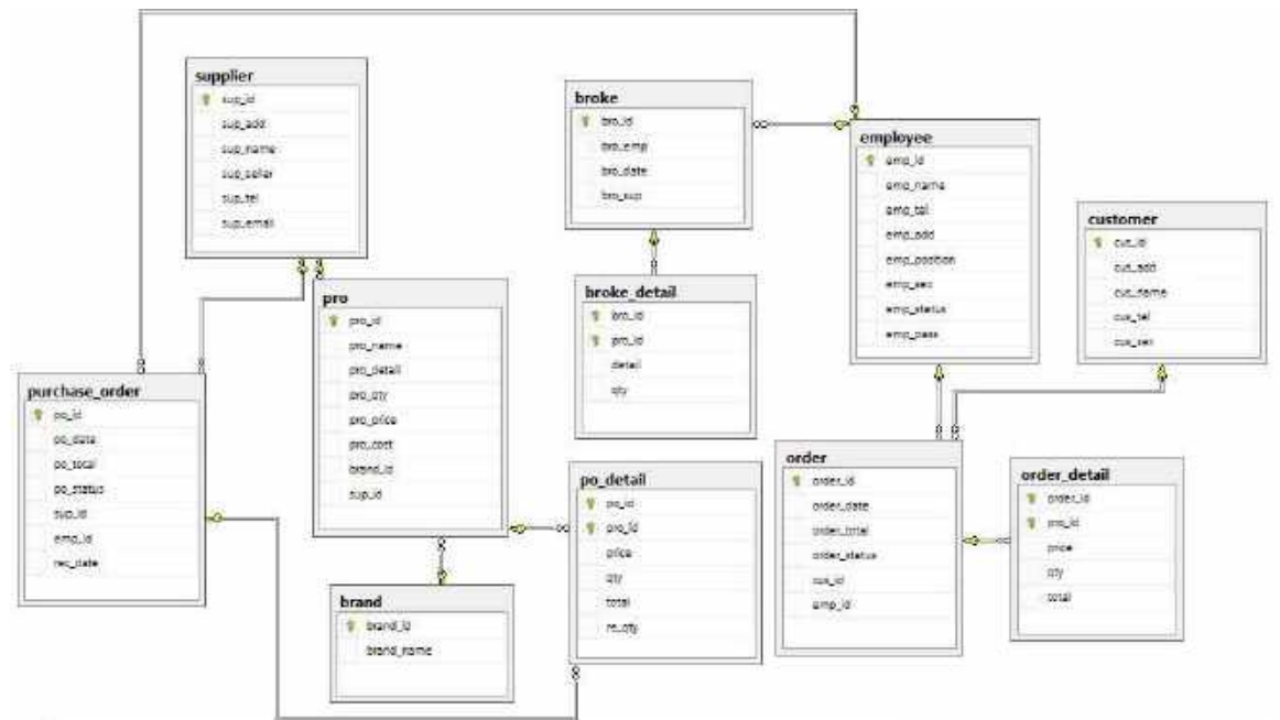
ภาพที่ 3.24 การแสดงความสัมพันธ์ของข้อมูล
