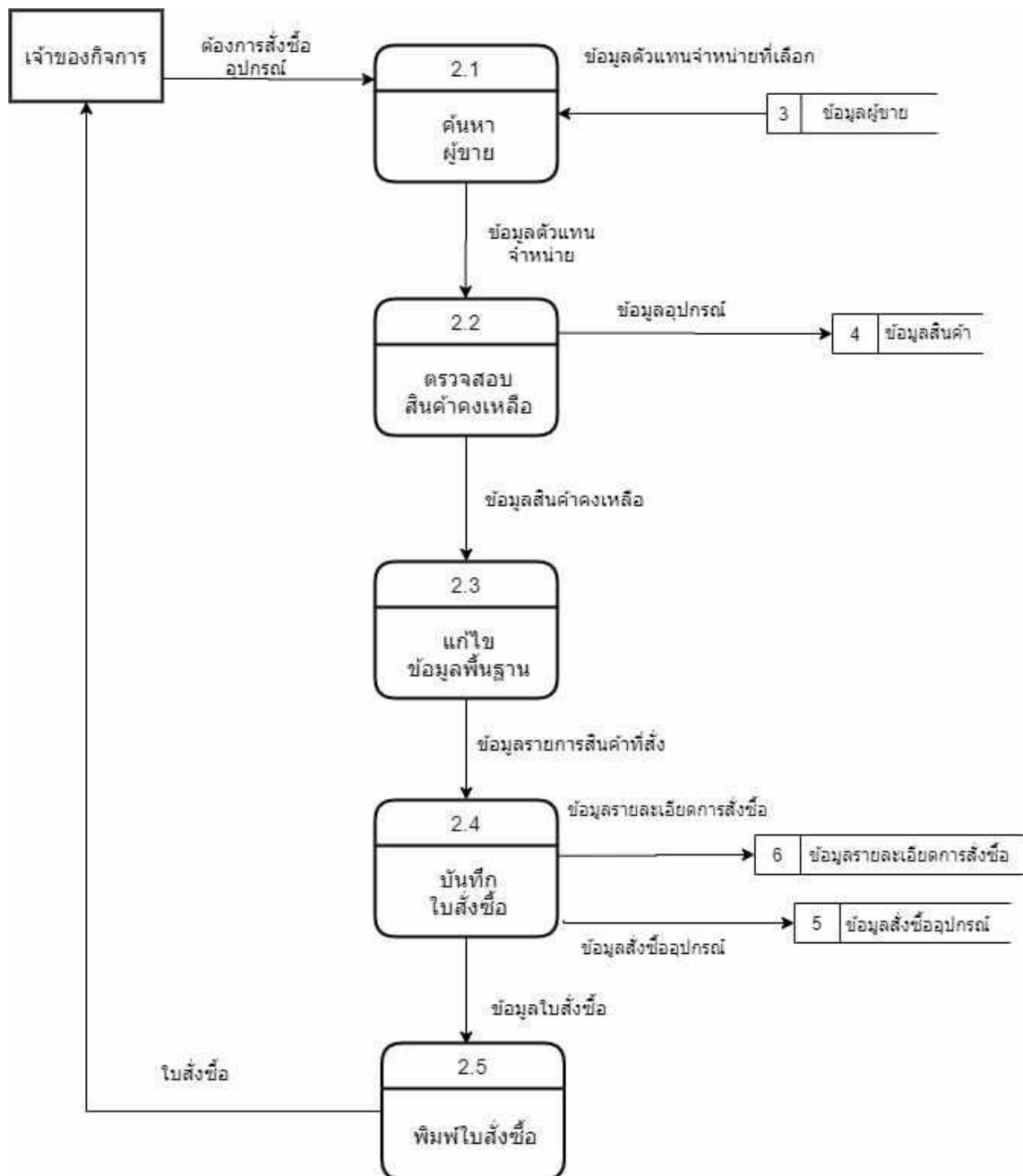
ภาพที่ ก.8 Data Flow Diagram Level 1 ของ Process 2: สั่งซื้อสินค้าอุปกรณ์
