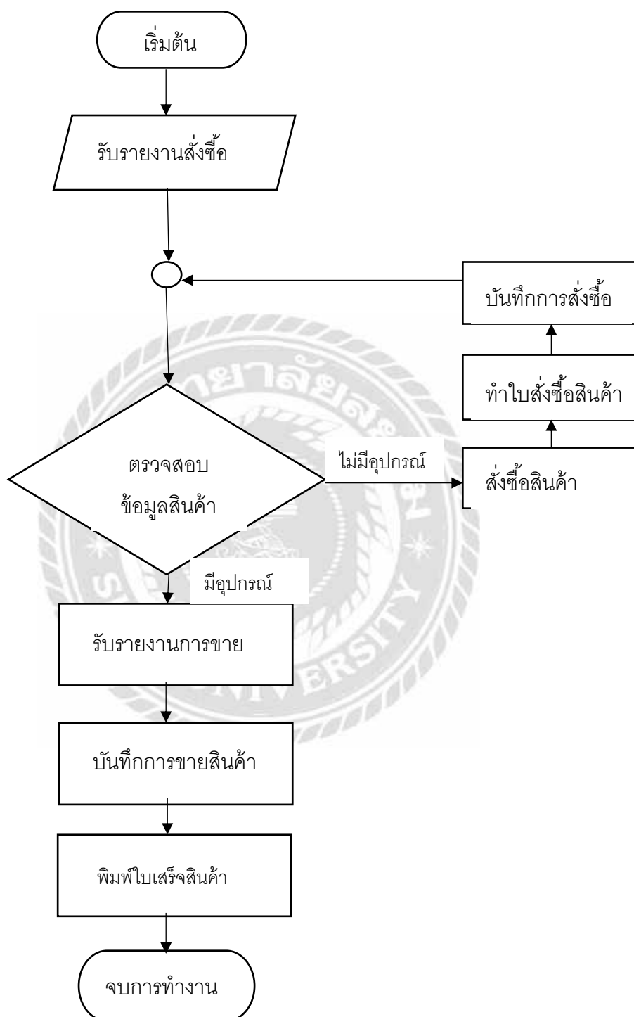
ภาพที่ 3.1 แผนผังการทำงานของระบบงานปัจจุบัน
