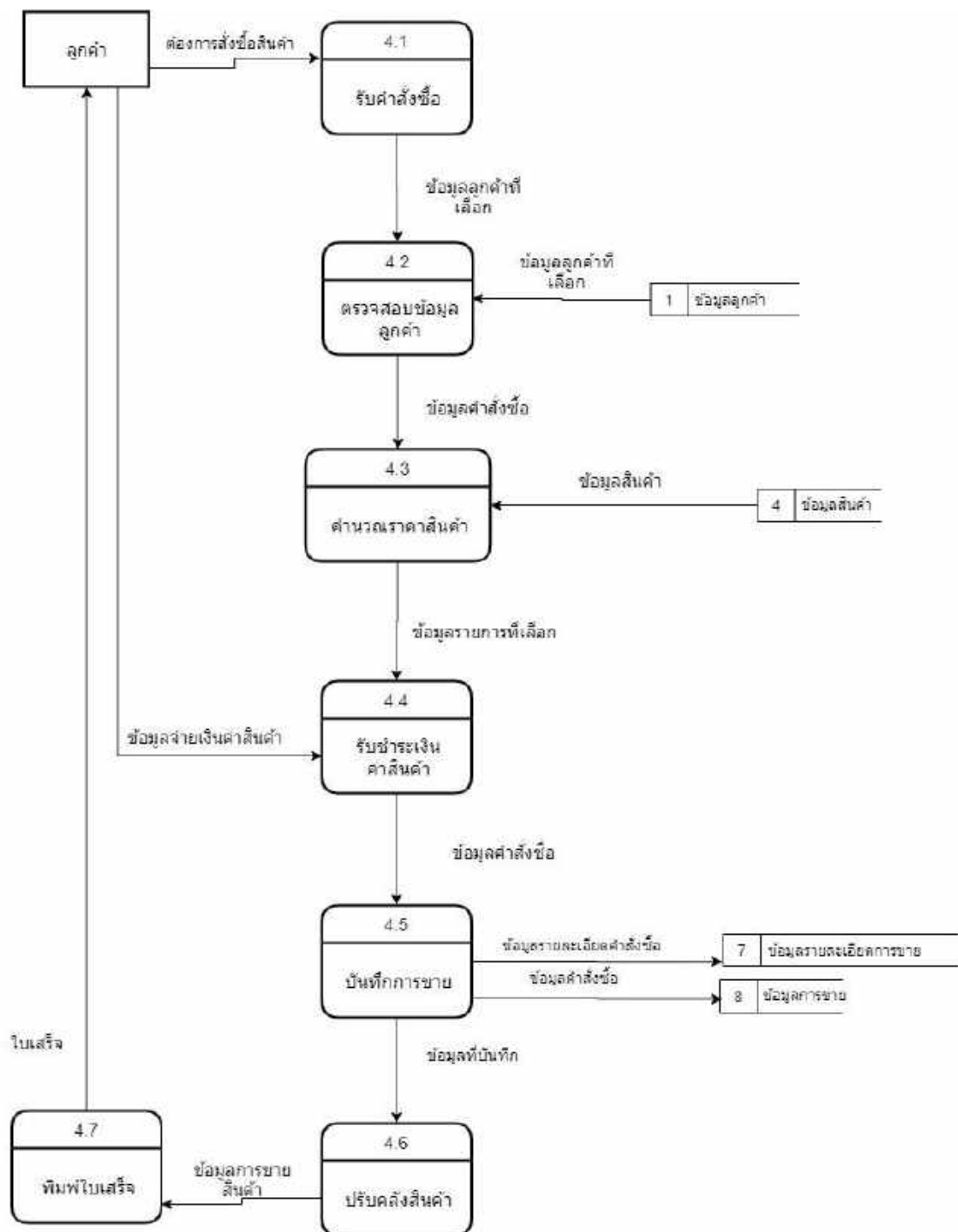
ภาพที่ ก.10 Data Flow Diagram Level 1 ของ Process 4: ขายสินค้า
