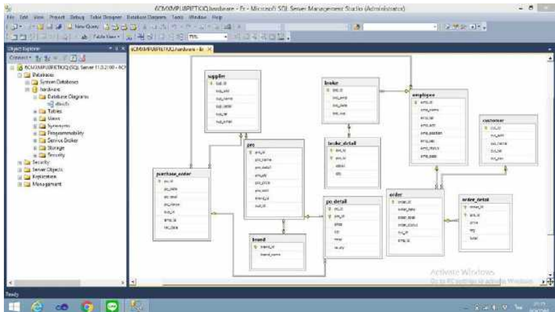
ภาพที่ 3.25 การออกแบบฐานข้อมูล
