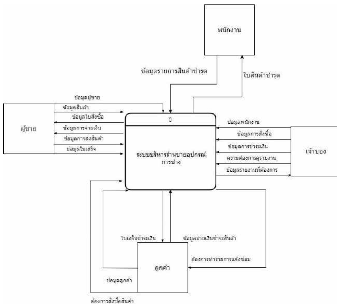
ภาพที่ ก.4 Context Diagram ระบบบริหารงานร้านขายอุปกรณ์การช่าง
