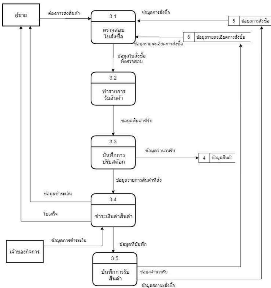
ภาพที่ ก.9 Data Flow Diagram Level 1 ของ Process 3: รับสินค้าอุปกรณ์
