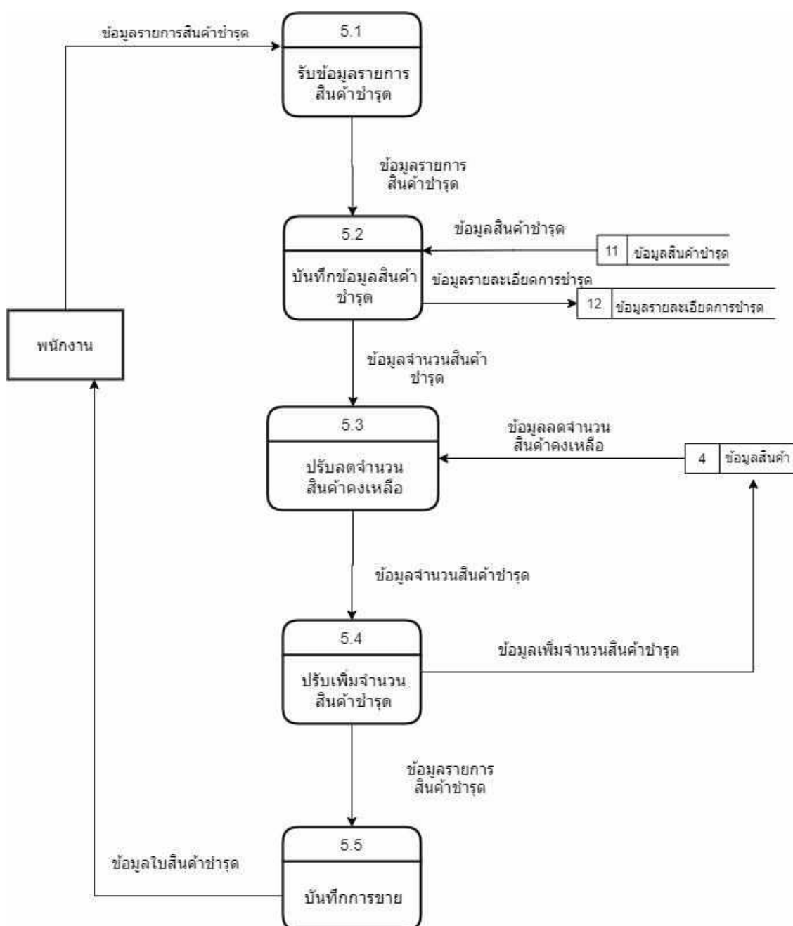
ภาพที่ ก.11 Data Flow Diagram Level 1 ของ Process 5: สินค้าชำรุด
