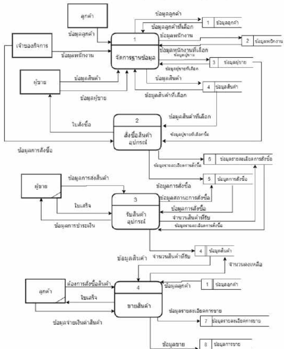
ภาพที่ ก.5 Data Flow Diagram Level 0 ระบบร้านขายอุปกรณ์การช่าง
