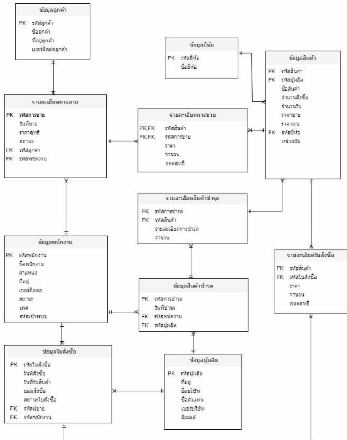
ภาพที่ ก.3 E-R Diagram (ภาษาไทย)
