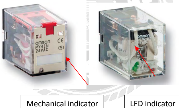
รูปที่ 2.10 Mechanical indicator , LED indicator
