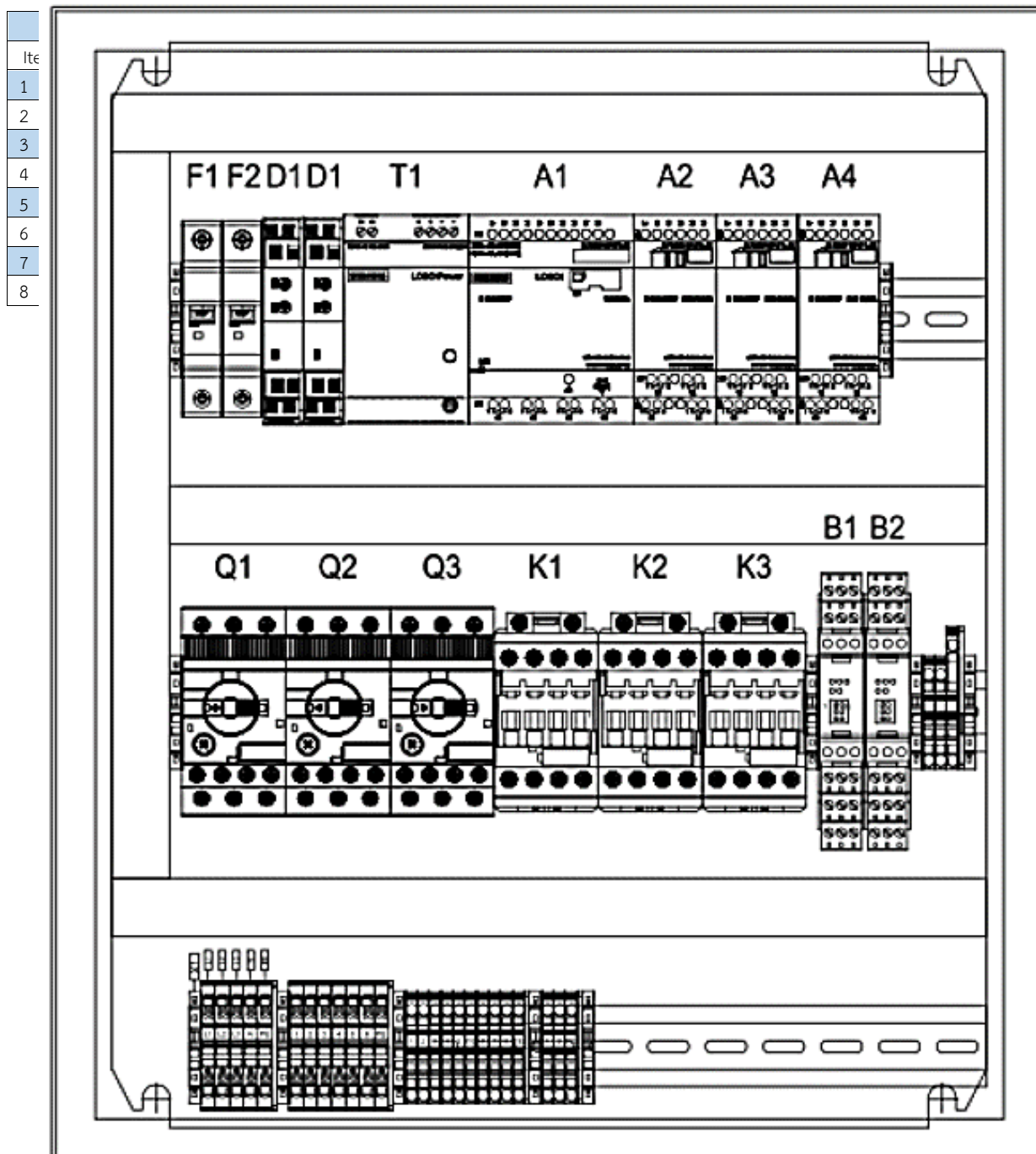
รูปที่ 4.10 รูปแสดงตัวอย่าง Layout อุปกรณ์ที่ติดตั้งภายในตู้ควบคุมไฟฟ้า
