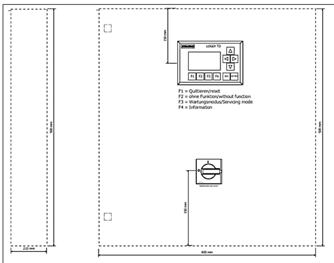
รูปที่ 4.14 รูปแสดงตัวอย่าง Layout ของอุปกรณ์ที่ติดตั้งด้านนอกของตู้ควบคุมไฟฟ้า
