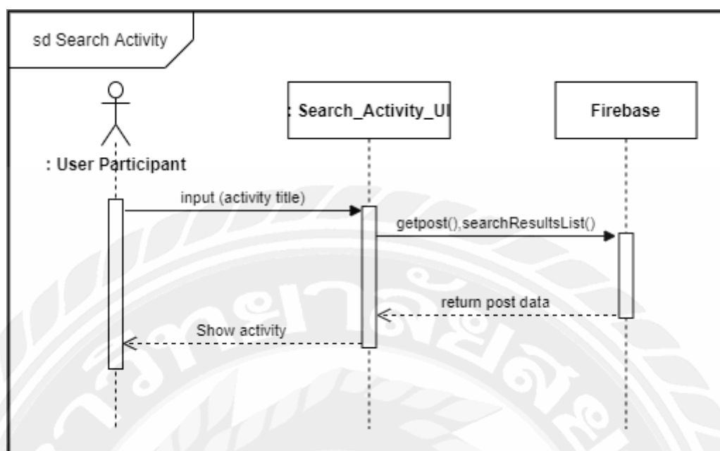
รูปที่ 3.8 Sequence diagram : Search Activity
