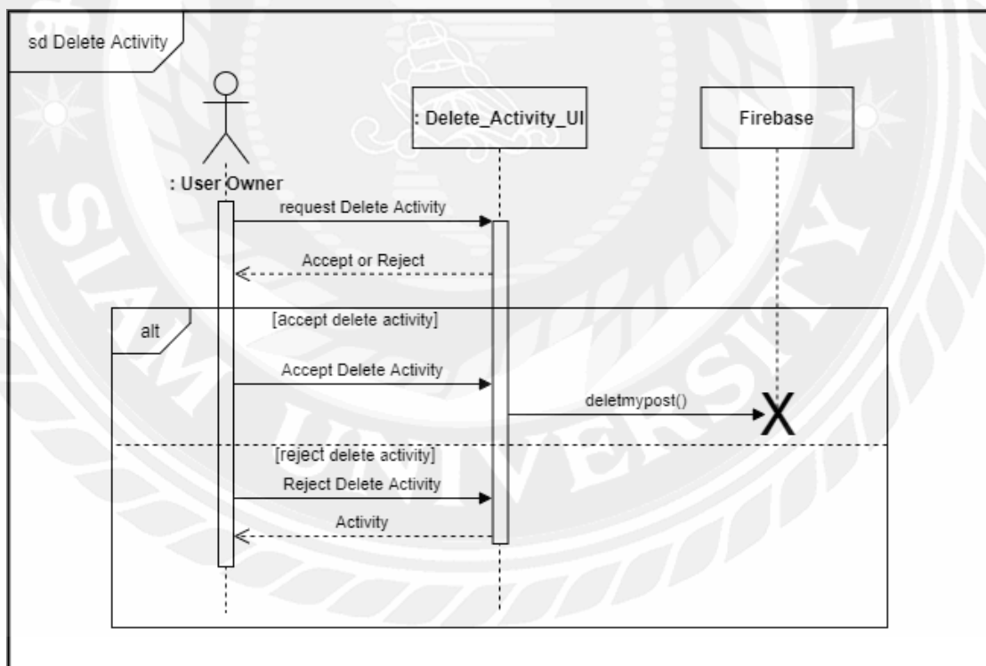
รูปที่ 3.7 Sequence diagram : Delete Activity
