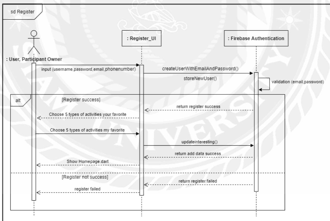
รูปที่ 3.3 Sequence diagram : Register
