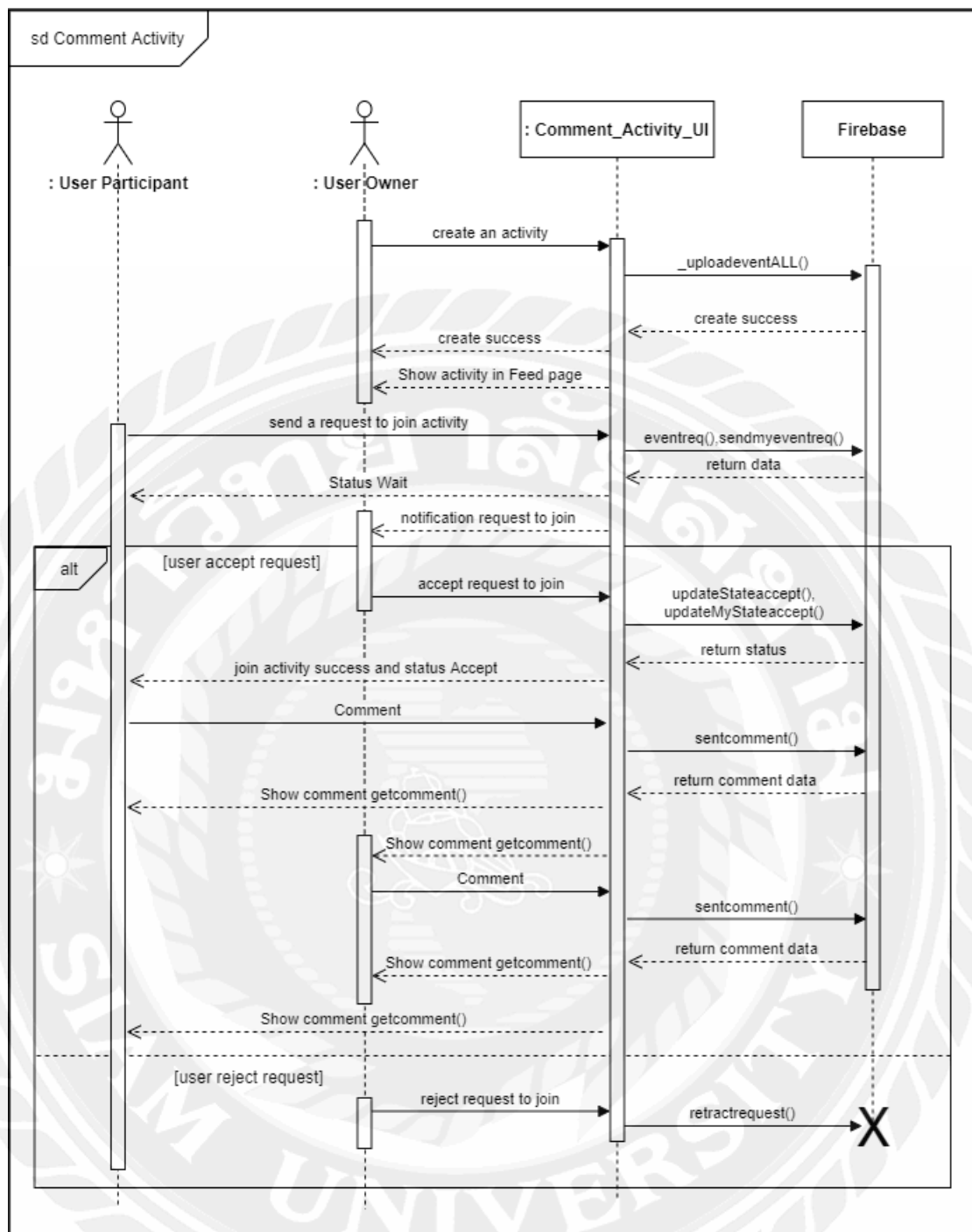
รูปที่ 3.11 Sequence diagram : Comment Activity
