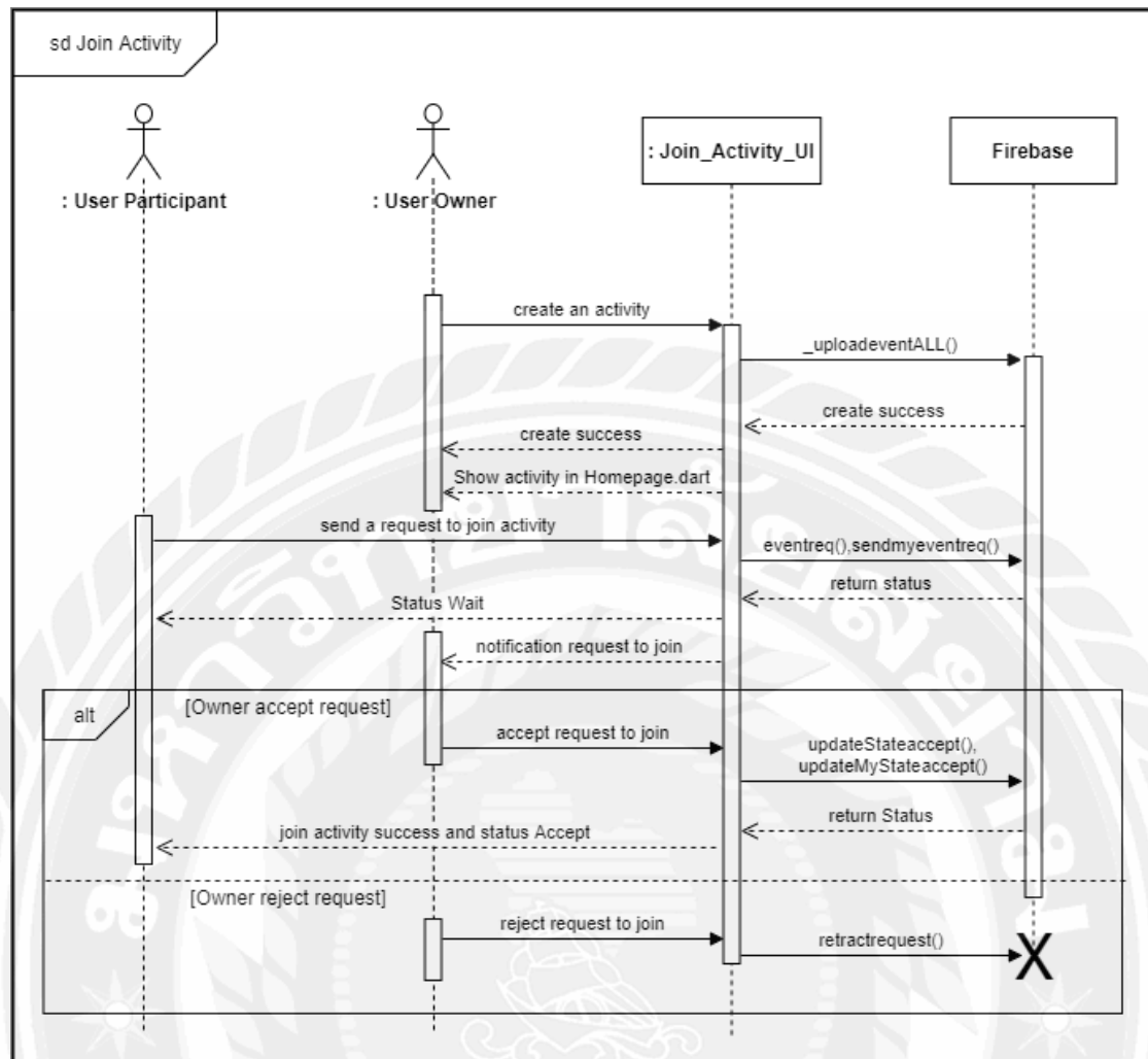
รูปที่ 3.10 Sequence diagram : Join Activity
