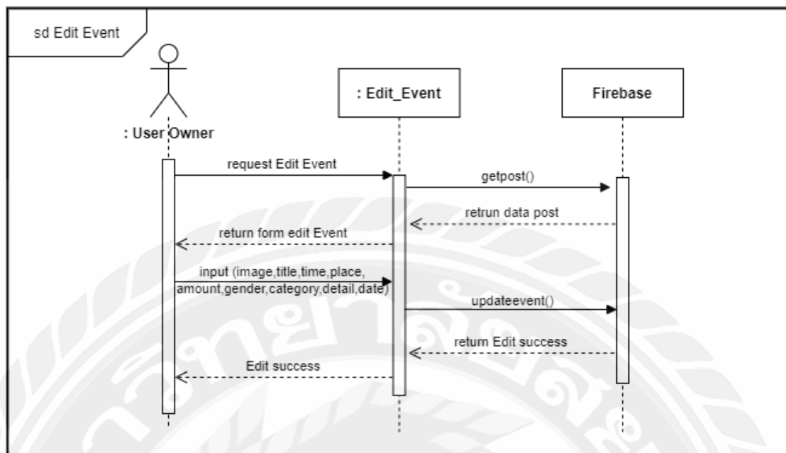
รูปที่ 3.6 Sequence diagram : Edit Event
