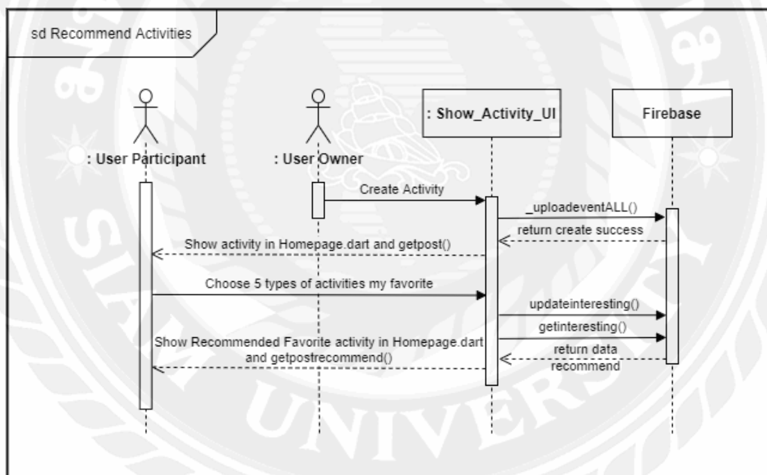
รูปที่ 3.15 Sequence diagram : Recommend Activities
