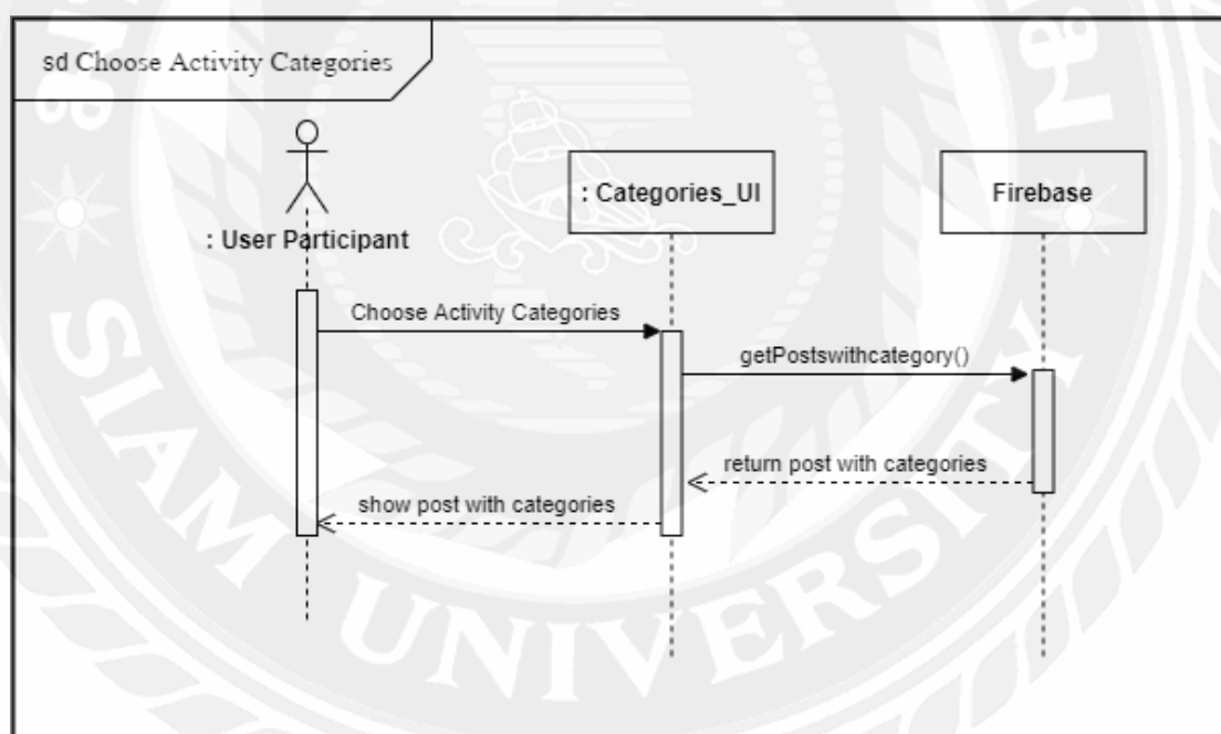
รูปที่ 3.9 Sequence diagram : Choose Activity Categories
