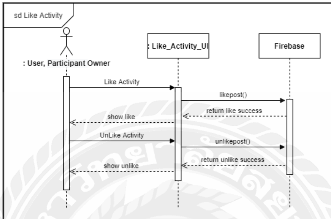
รูปที่ 3.12 Sequence diagram : Like Activity
