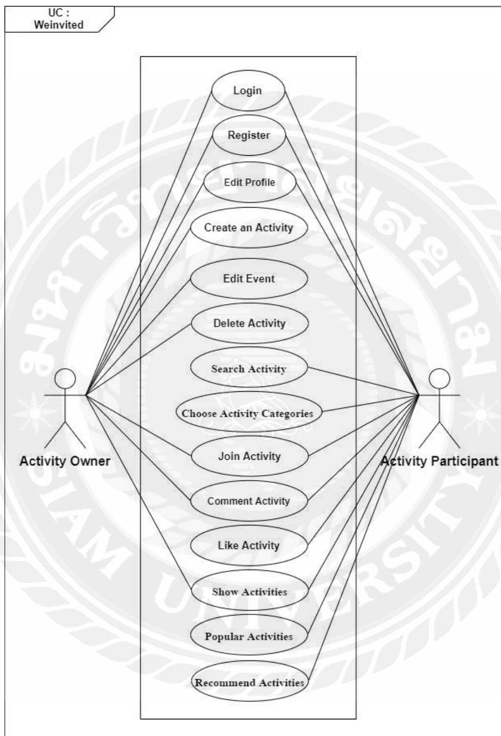
รูปที่ 3.1 Use Case Diagram ของแอปพลิเคชัน We Invited
