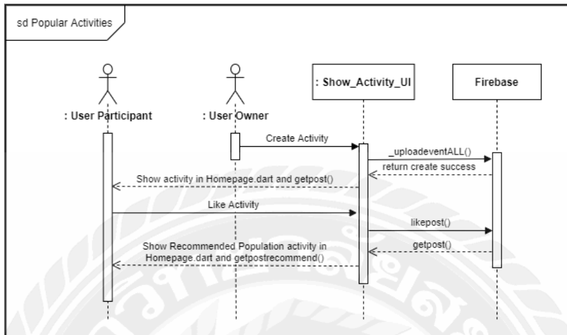
รูปที่ 3.14 Sequence diagram : Popular Activities
