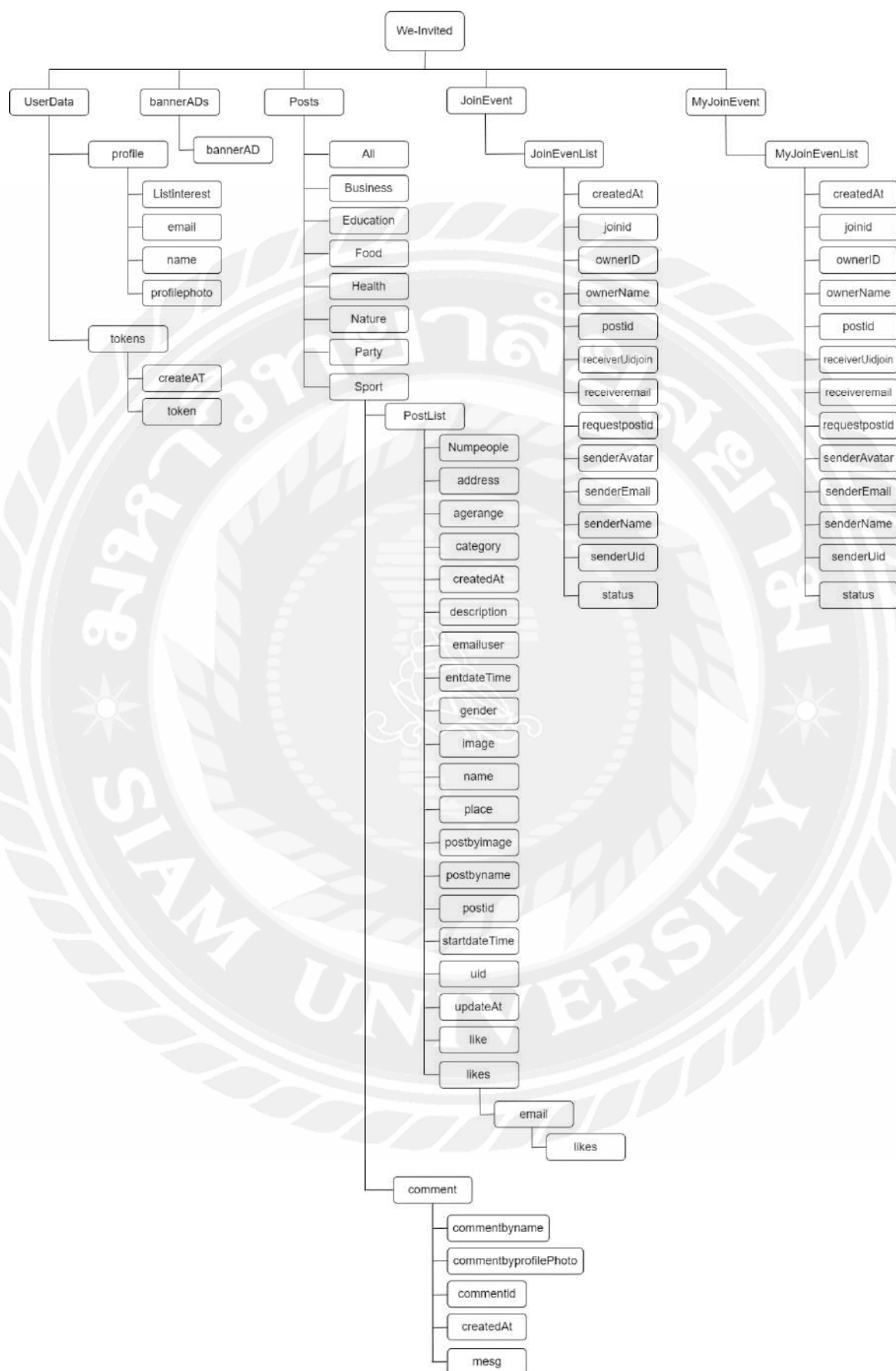
รูปที่ 3.17 โครงสร้างของข้อมูล (NoSQL Structure)
