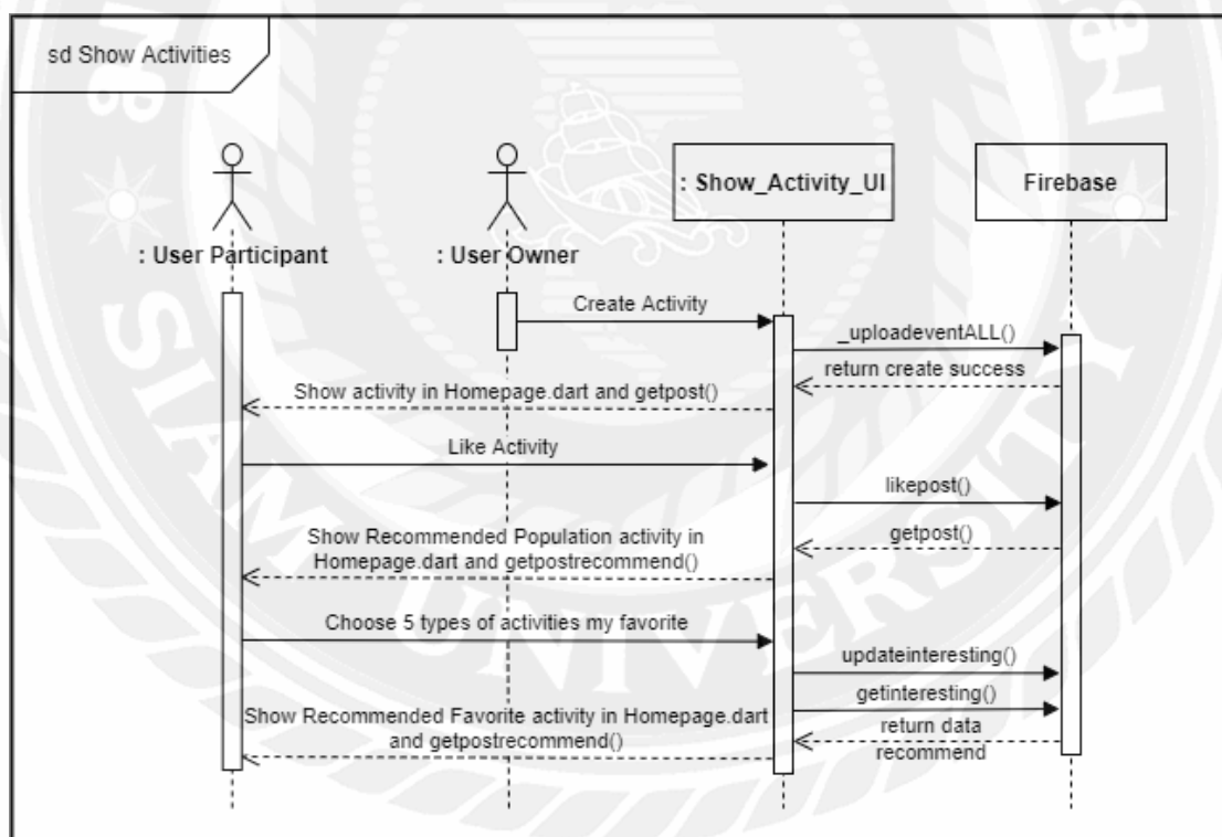
รูปที่ 3.13 Sequence diagram : Show Activities
