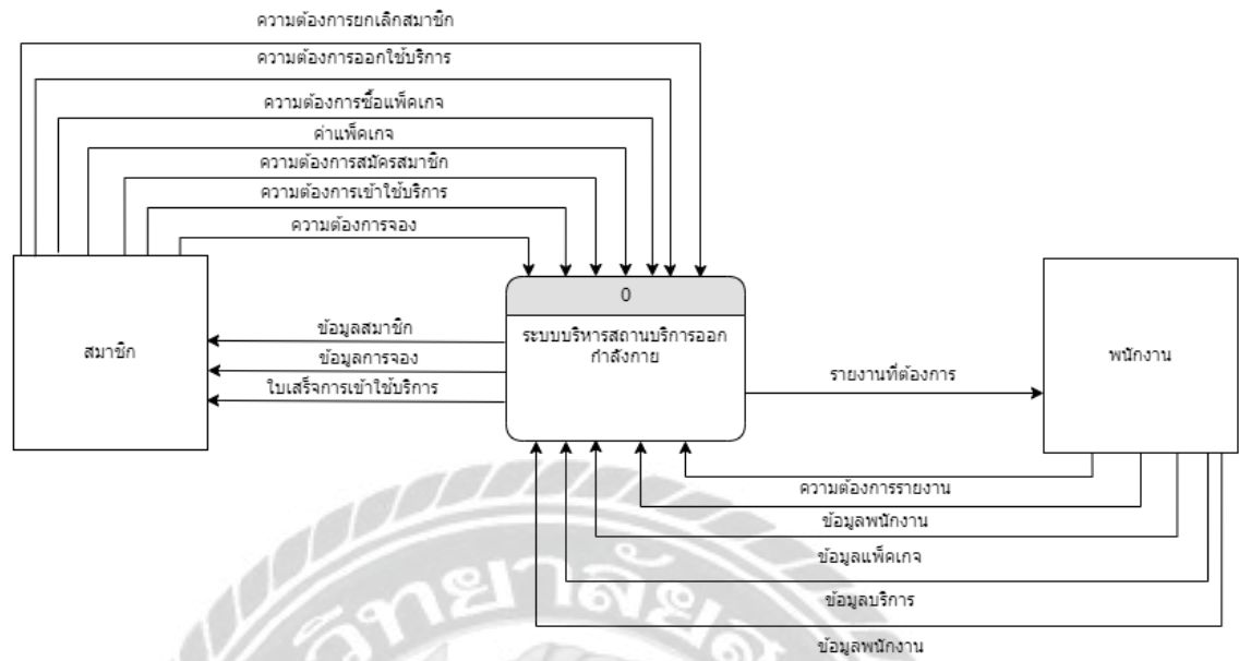
ภาพที่ ก.4 Context Diagram ระบบบริหารสถานบริการออกกำลังกาย
