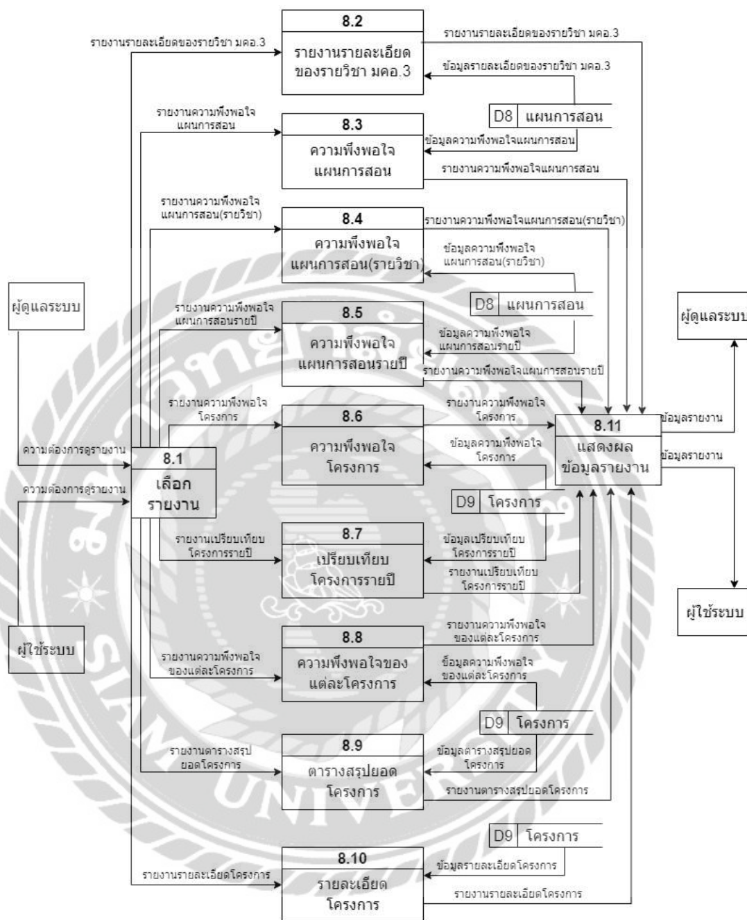
ภาพที่ ก.13 Data Flow Diagram Level 1 Process 8 ออกรายงาน
