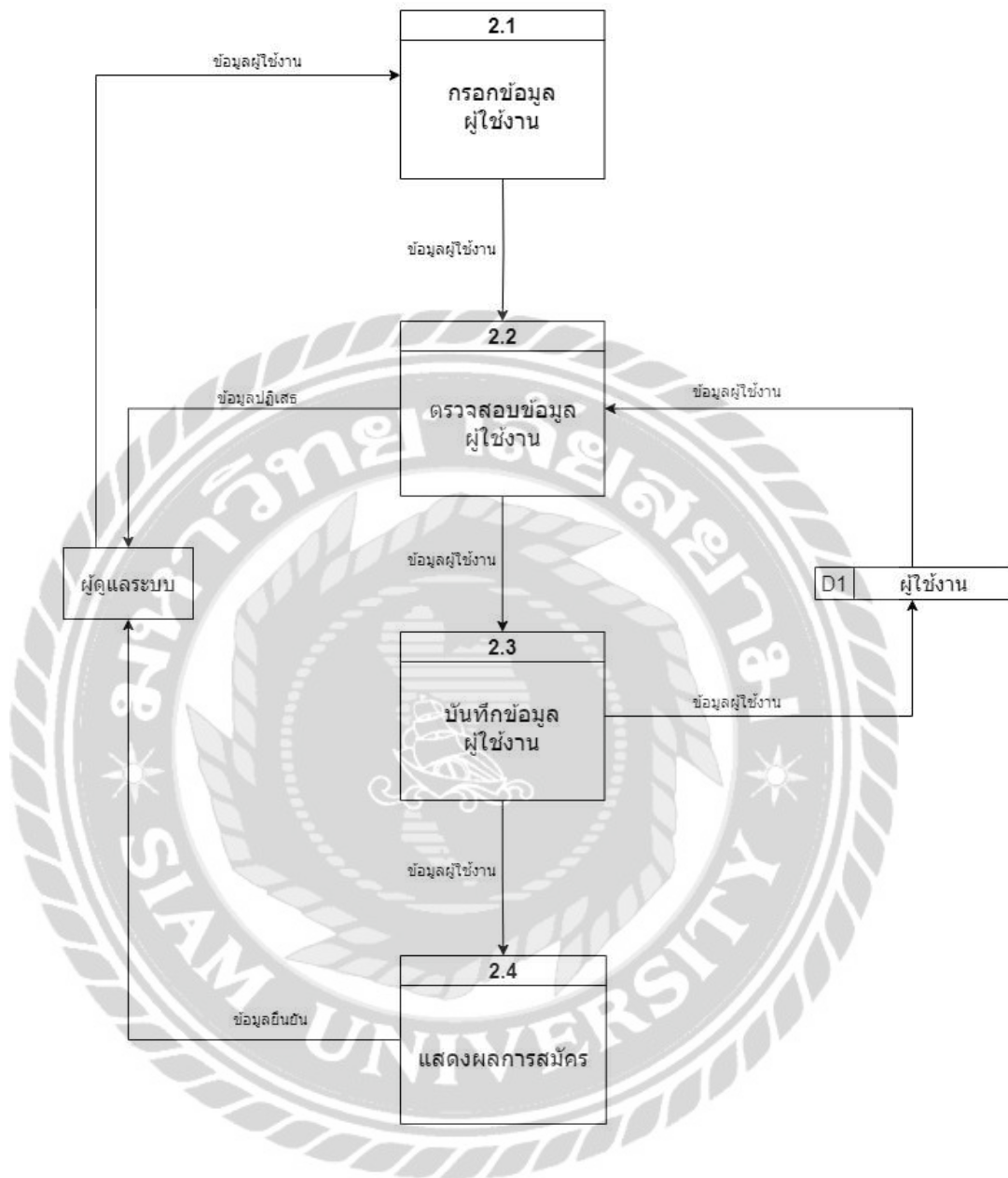
ภาพที่ ก.7 Data Flow Diagram Level 1 Process 2 สมัครงาน
