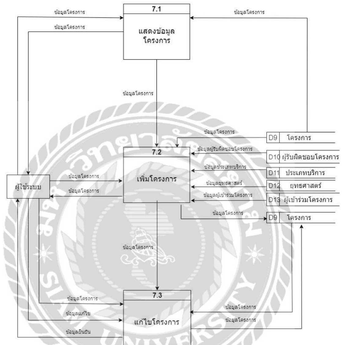
ภาพที่ ก.12 Data Flow Diagram Level 1 Process 7 จัดการโครงการ
