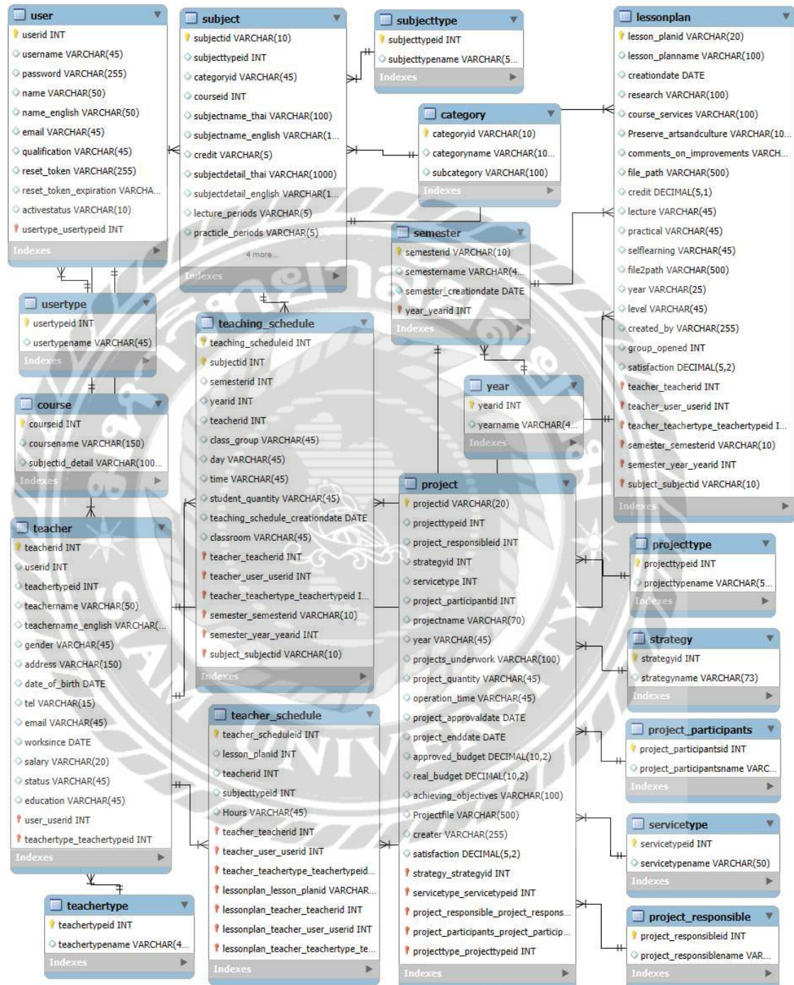
ภาพที่ 3.60 การแสดงความสัมพันธ์ของข้อมูล
