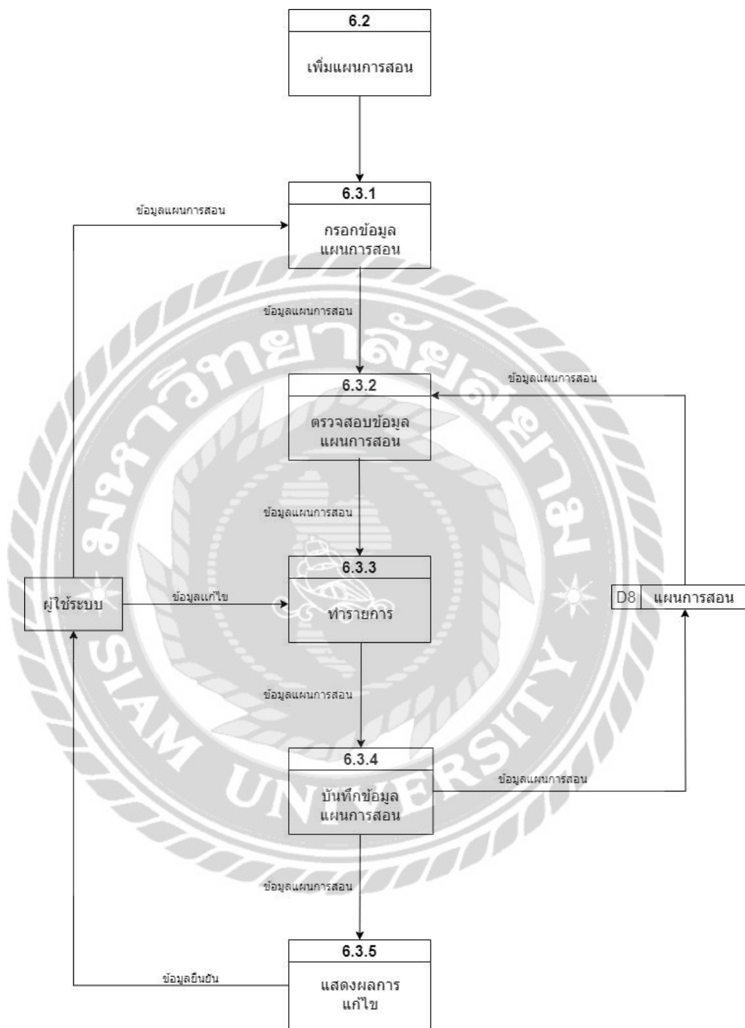
ภาพที่ ก.15 Data Flow Diagram Level 2 Process 6.3 แก้ไขแผนการสอน
