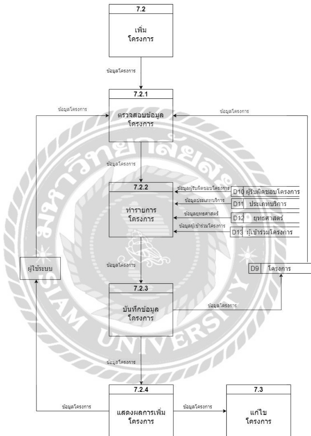
ภาพที่ ก.16 Data Flow Diagram Level 2 Process 7.2 เพิ่มโครงการ
