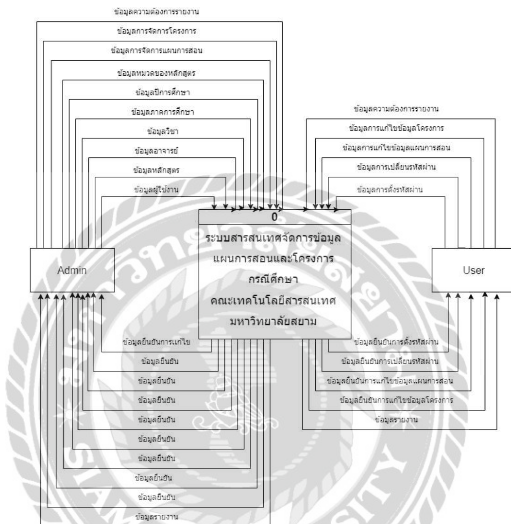
ภาพที่ ก.4 Context Diagram ระบบสารสนเทศจัดการข้อมูลแผนการสอนและโครงการ กรณีศึกษา คณะเทคโนโลยีสารสนเทศ มหาวิทยาลัยสยาม
