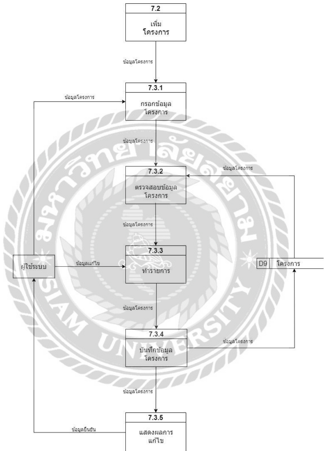
ภาพที่ ก.17 Data Flow Diagram Level 2 Process 7.3 แก้ไขโครงการ
