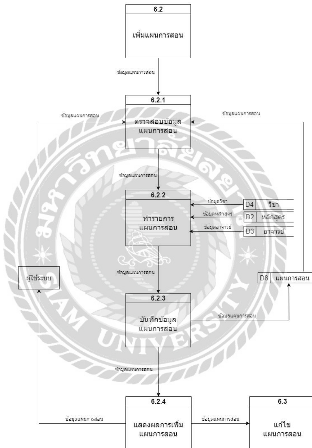
ภาพที่ ก.14 Data Flow Diagram Level 2 Process 6.2 เพิ่มแผนการสอน
