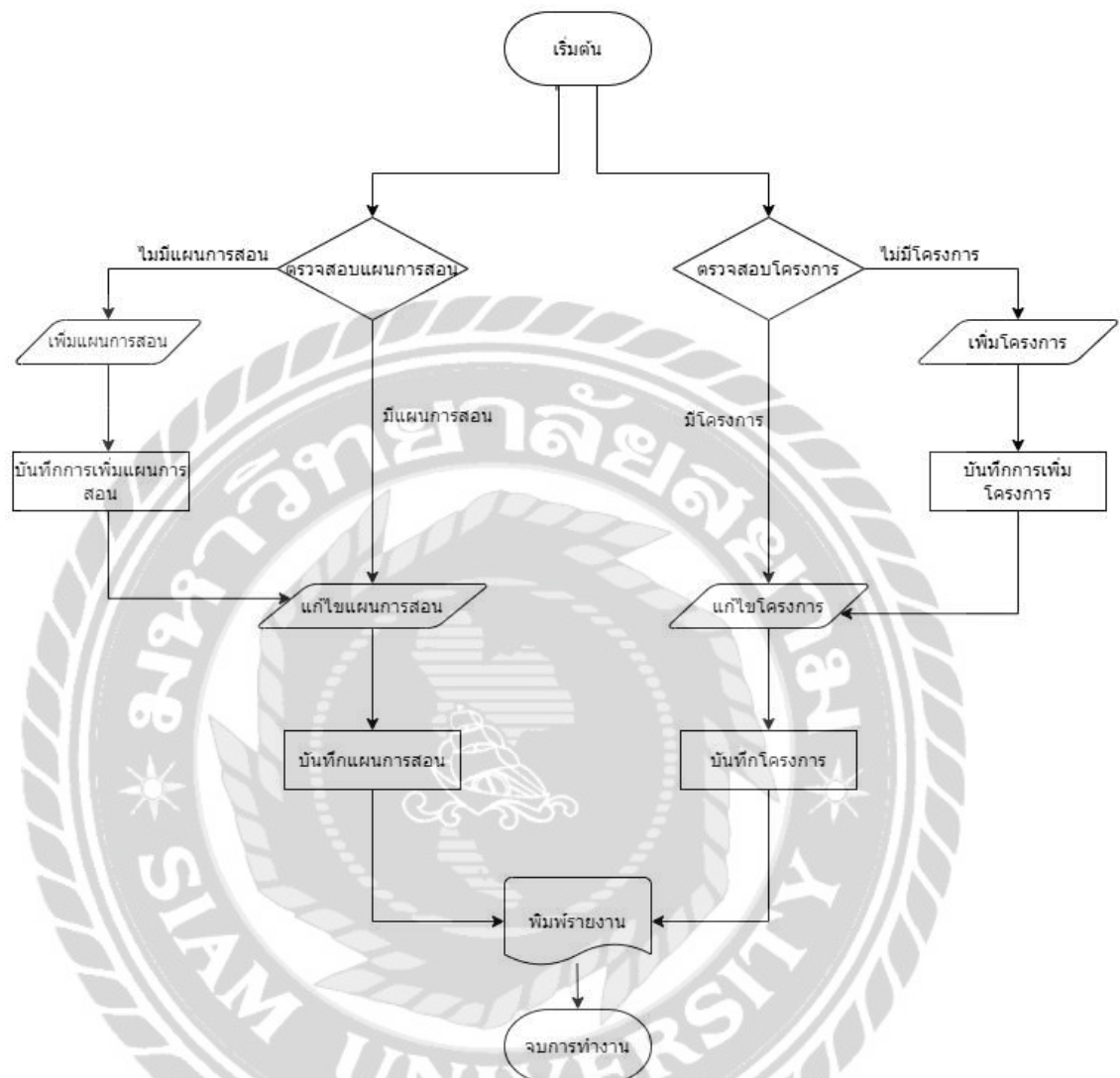
ภาพที่ 3.1 แผนผังการทำงานของระบบงานปัจจุบัน
