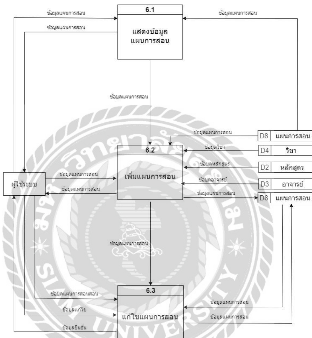
ภาพที่ ก.11 Data Flow Diagram Level 1 Process 6 จัดการแผนการสอน
