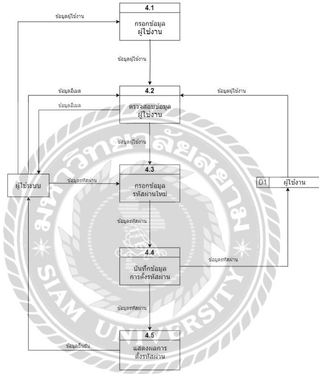
ภาพที่ ก.9 Data Flow Diagram Level 1 Process 4 ลืมรหัสผ่าน
