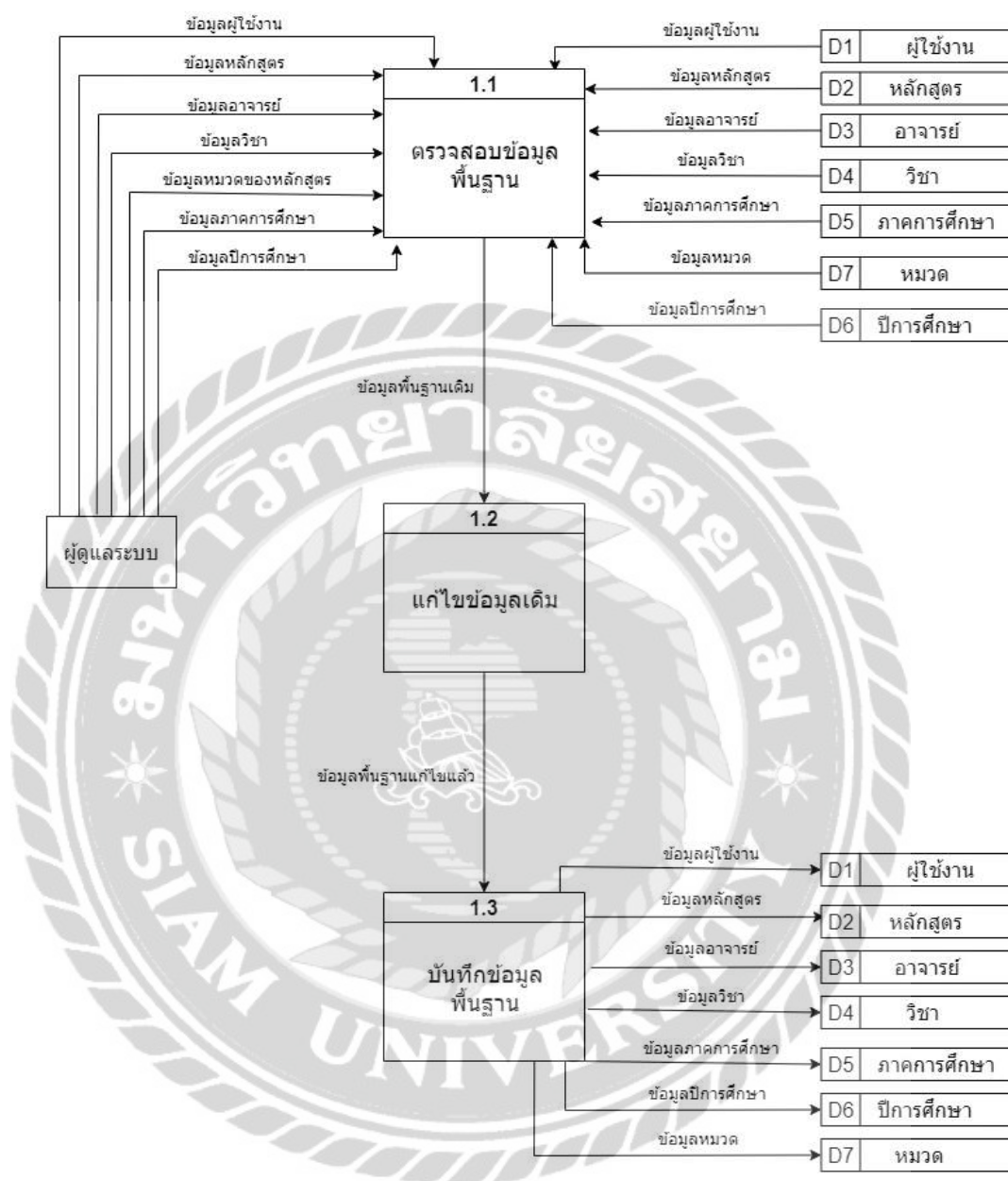
ภาพที่ ก.6 Data Flow Diagram Level 1 Process 1 จัดการข้อมูลพื้นฐาน
