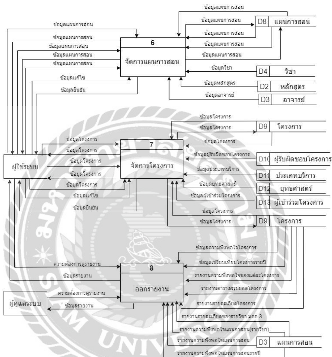
ภาพที่ ก.5 Data Flow Diagram Level 0 (ต่อ) ระบบสารสนเทศจัดการข้อมูลแผนการสอนและโครงการ วิทยาลัยเทคโนโลยีสารสนเทศ มหาวิทยาลัยสยาม
