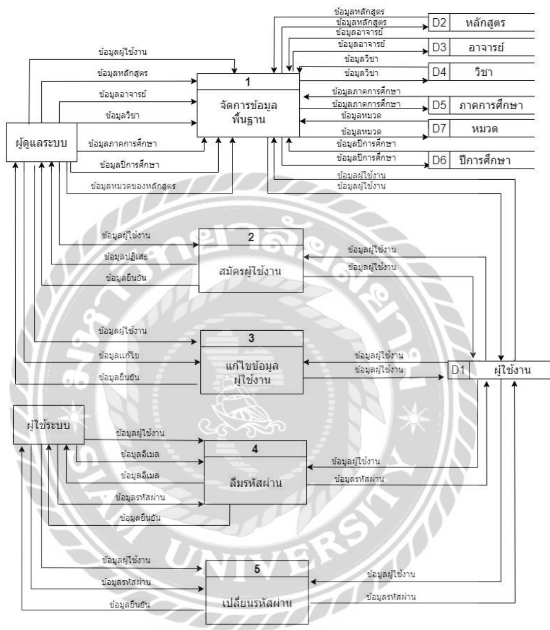
ภาพที่ ก.5 Data Flow Diagram Level 0 ระบบสารสนเทศจัดการข้อมูลแผนการสอนและโครงการ กรณีศึกษาคณะเทคโนโลยีสารสนเทศ มหาวิทยาลัยสยาม
